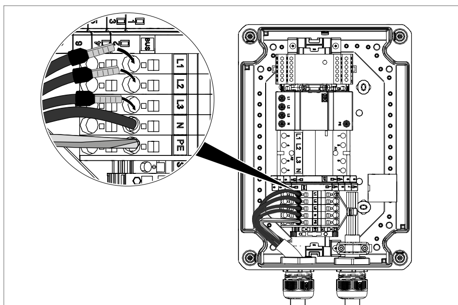
Ábra 9: A tápkábel csatlakoztatása
