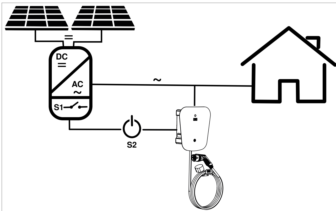
Ábra 2: Statikus, napelemes rendszerre optimalizált töltés alkalmazási példája
