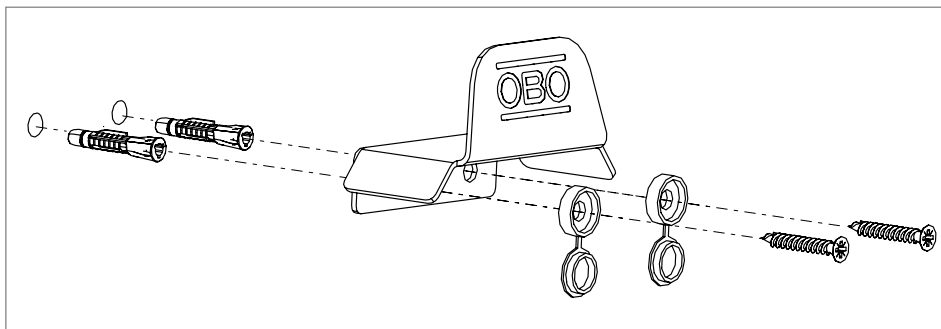
Ábra 14: A kábeltartó felszerelése
