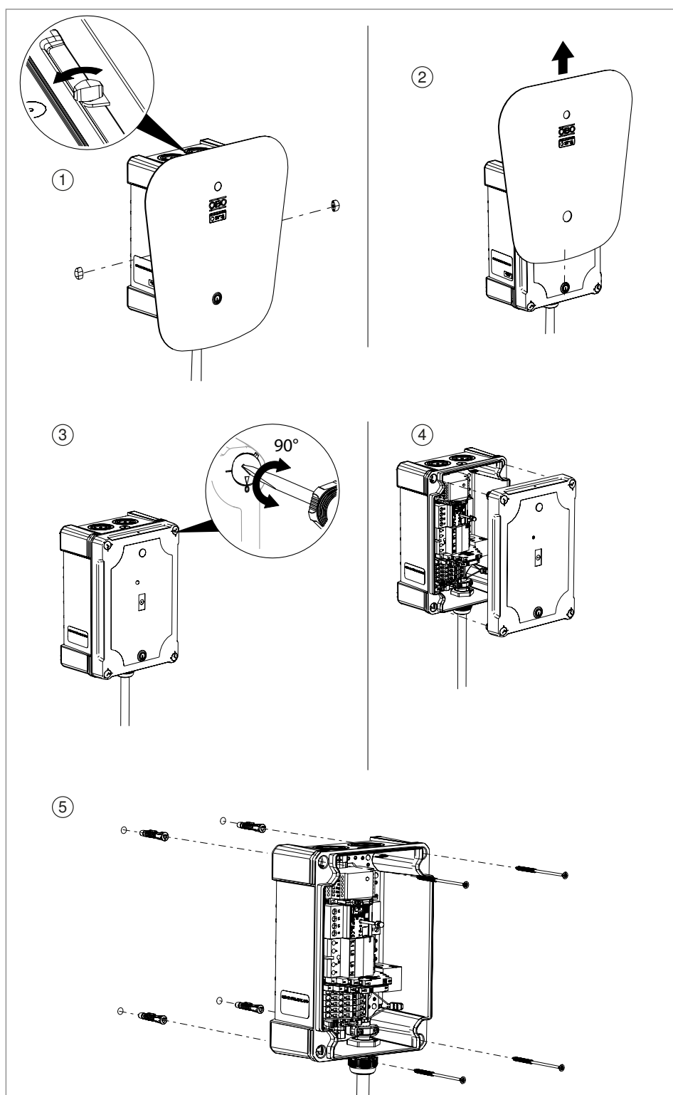
Ábra 6: Az előlap eltávolítása
