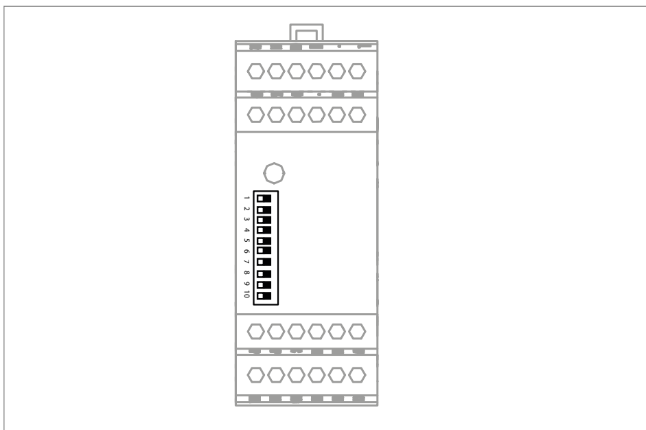
Ábra 15: A DIP-kapcsoló konfigurálása
