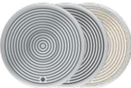
R9-es névleges méret, alumínium Külső méret: Ø 325 mm, 12 x Modul 45
